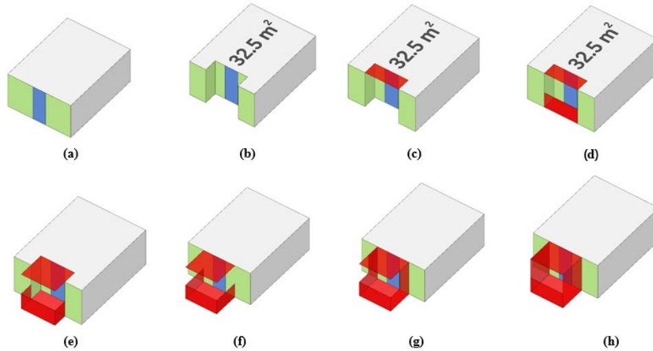
Gambar 4 Warna hijau : dinding eksterior , Merah : balkon, biru : kaca ; (a) Baseline (b) Bentuk, (c) Shading Horizontal , (d) Full Balkon, (e) Balkon Semi Luar, (f) Balkon Luar, (g) Balkon Kombinasi Semi Luar , (h) Balkon Kombinasi Dalam
