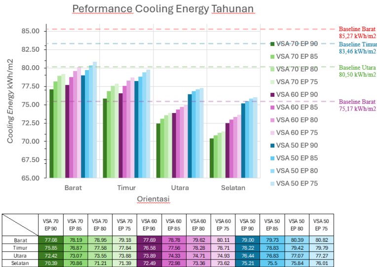
Gambar 8 Cooling Energy per Bulan (Maret) pada Empat Orientasi
