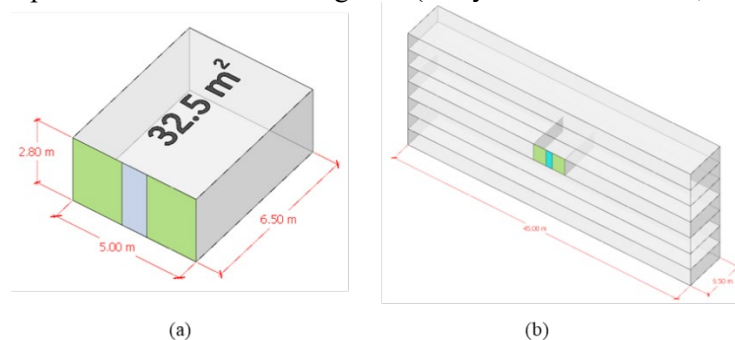
Gambar 2 (a) Detail Ukuran Ruang Uji (b) Lokasi tempat unit pada hunian vertikal
