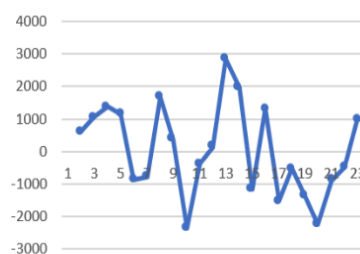
Gambar 4. Verifikasi Moving Range
