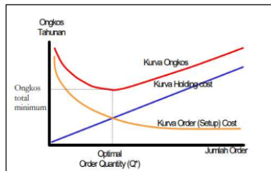
Gambar 3 Grafik EOQ
