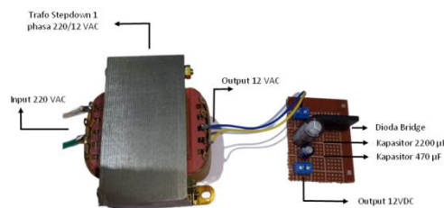
Gambar 4. Catu Daya
