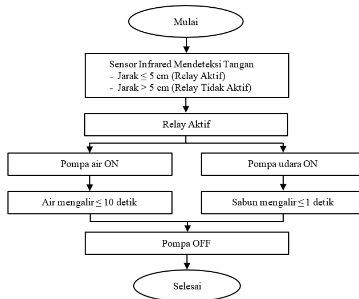
Gambar 2. Diagram Alur Pengujian Alat
