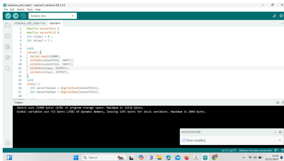
Gambar 17. Verifikasi Program Pada Arduino IDE
